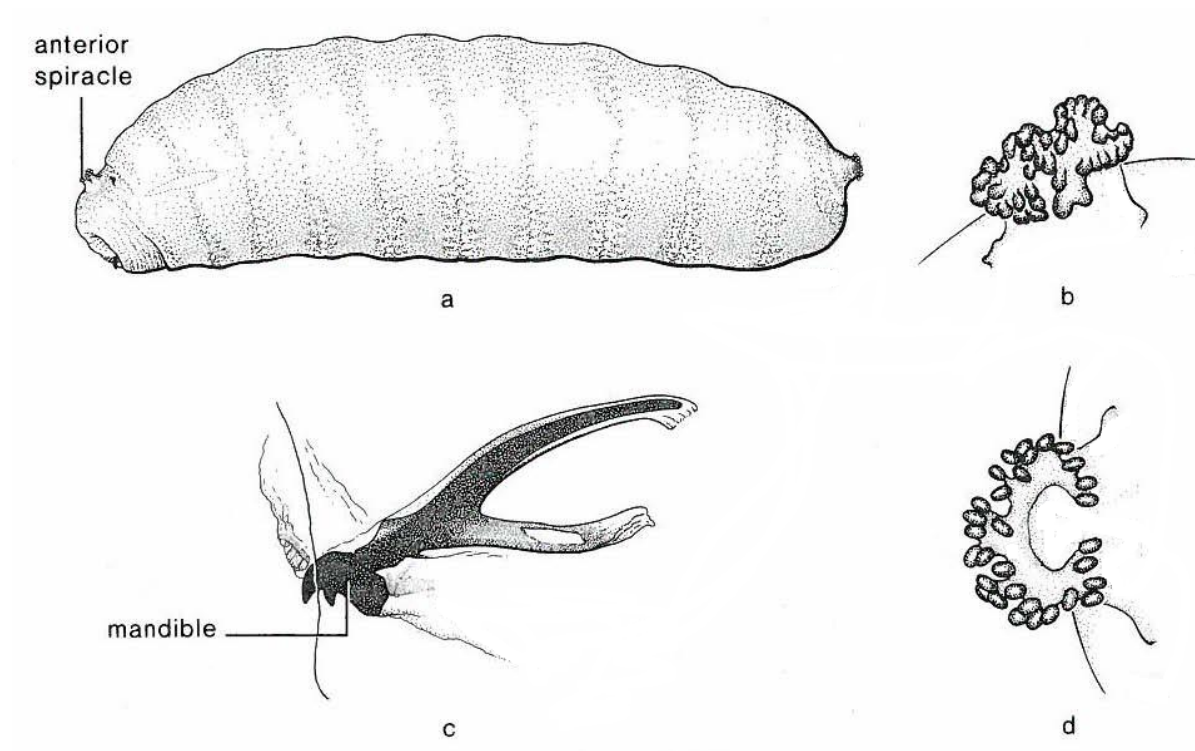
Figure 8. Larval morphology of Agromyzidae ( Phytomyza chelonei ): (a) lateral view; (b) anterior spiracle; (c) cephalopharyngeal skeleton; and (d) posterior spiracle. Source: Stehr (1991).
